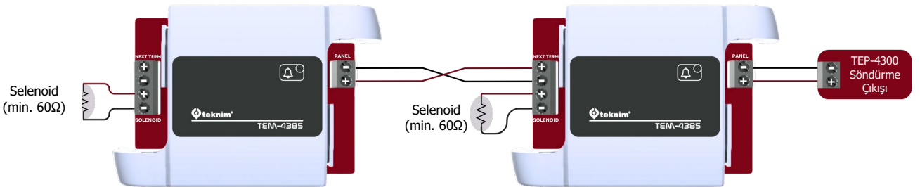
Şekil 3 - İki selenoid için bağlantı
